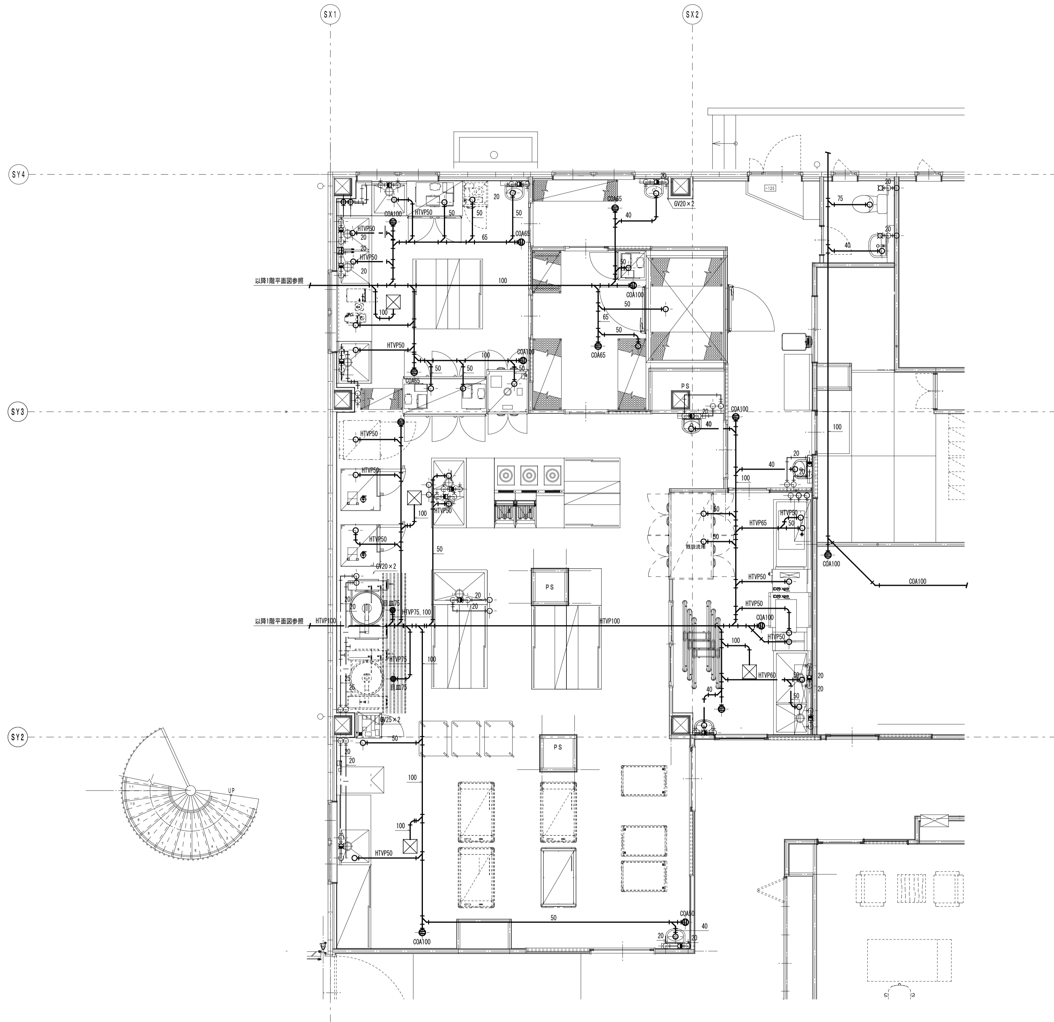
1階廚房平面詳細圖 S=1:50
